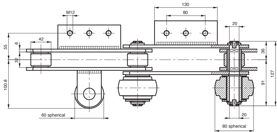
Chain P. 200x32x42 øR
