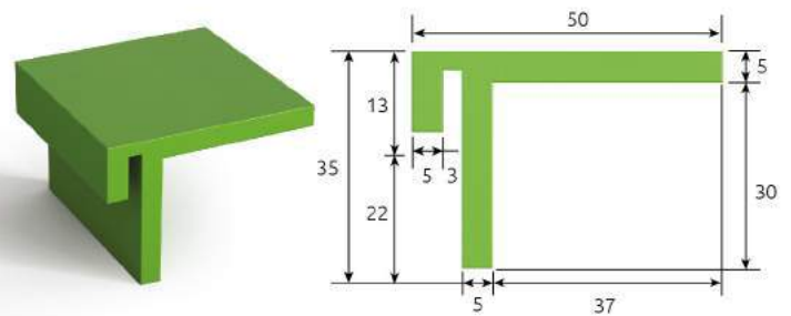
PERFILES INFERIOR PARA CURVA PCS-40 LN* LOWER PROFILE FOR PCS-40 LN* CURVE PROFIL INFERIEURE POUR COURBE PCS-40 LN*
