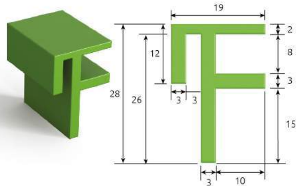
PERFILES SUPERIOR PARA CURVA PCS 26 LN* UPPER PROFILE FOR PCS-26 LN* CURVE PROFIL SUPERIEURE POUR COURBE PCS-26 LN*
