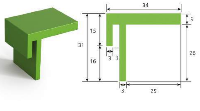
PERFILES INFERIOR PARA CURVA PCS-26 LN* LOWER PROFILE FOR PCS-26 LN* CURVE PROFIL INFERIEURE POUR COURBE PCS-26 LN*
